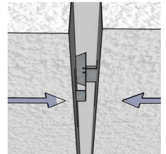
Zasunutie druhého panelu
