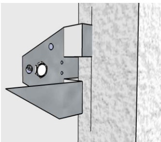
Upevnenie bočnej kotvy o stenu a napichnutie panelu.
