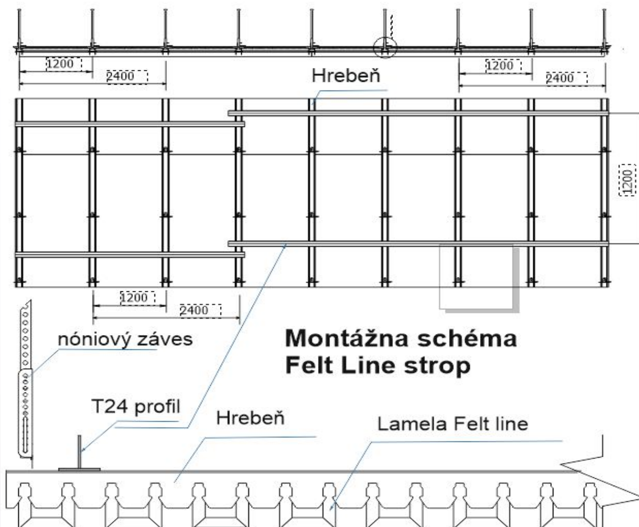
Zasúvanie lamiel do hrebeňov
